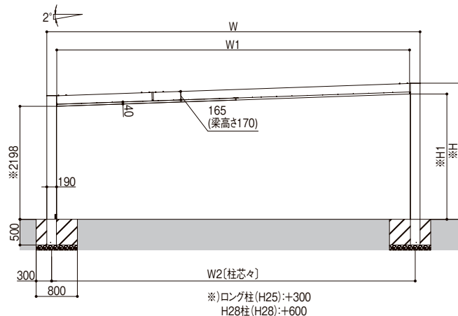
基本 正面図
