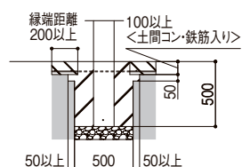
正面図
