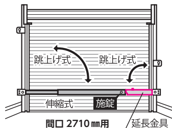
間口 2710 mm用
