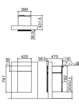
壁埋め込み仕様
