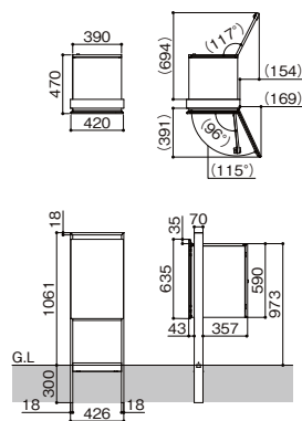
ボール建て仕様(埋め込み)
