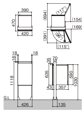
ボール建て仕様(ベース)
