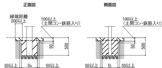
土間コンクリート併用基礎
