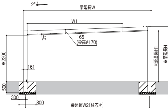
2本梁延長 W≤60 正面図
