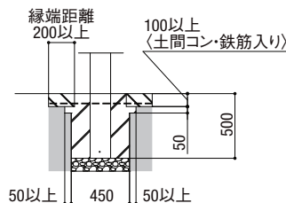
正面図
