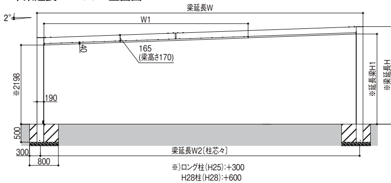
2本梁延長 W>60 正面図
