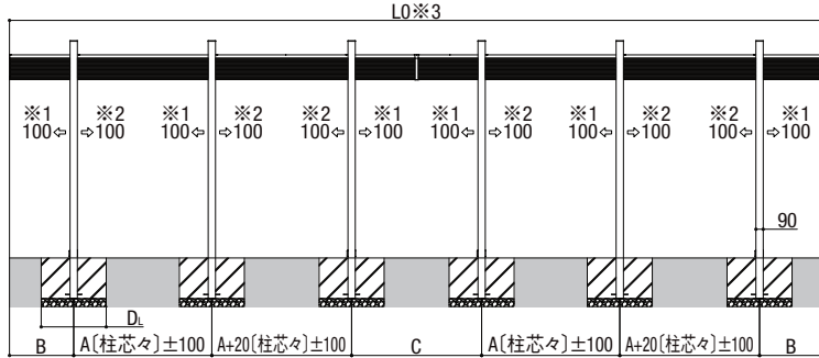
縦2連棟(W:48~60型) 側面図
