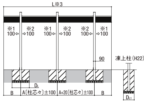
基本(W:48~60型) 側面図
