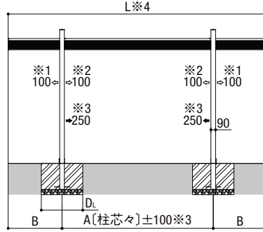
基本(W:48~60型) 側面図
