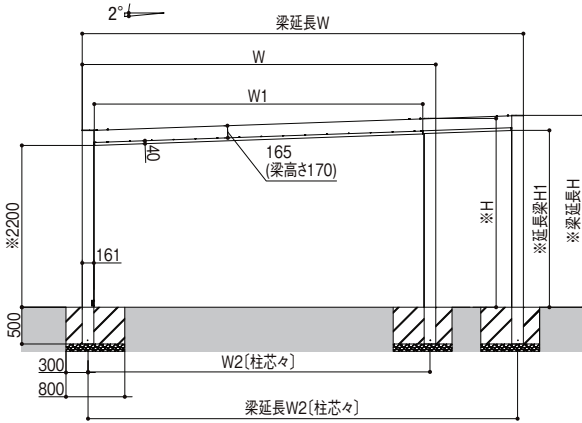
1本梁延長 W≤60 正面図
