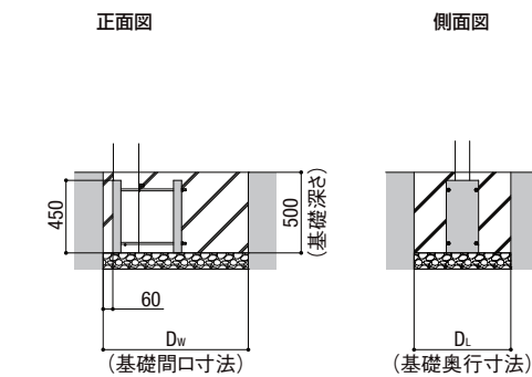
偏芯基礎
