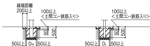
正面図
