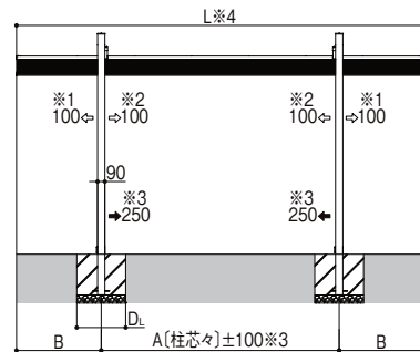
2本梁延長 側面図
