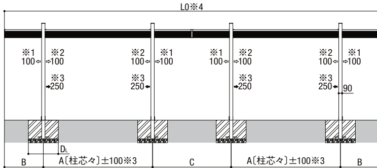
縦2連棟(W:48~60型) 側面図
