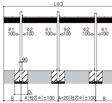
1・2本梁延長 側面図
