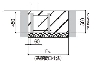
正面図
