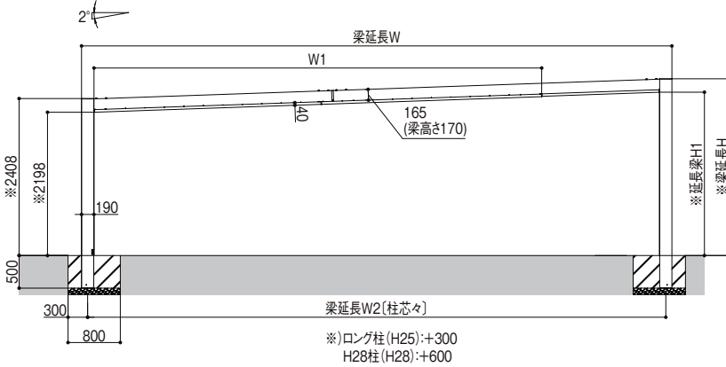
3本梁延長 正面図
