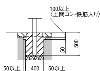
側面図
