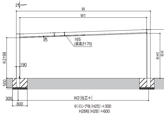
基本 正面図
