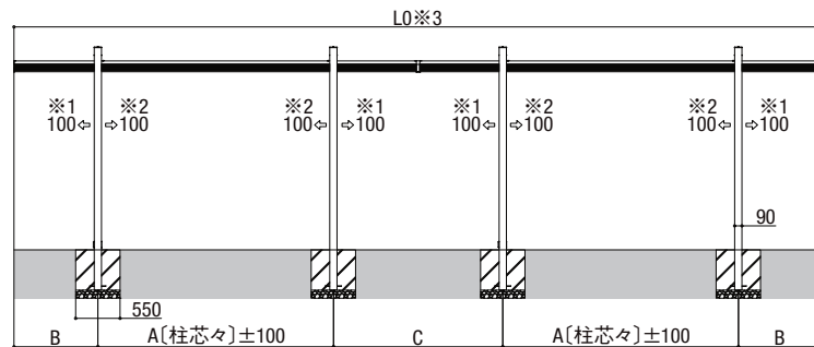
縦2連棟(W:30・33型) 側面図
