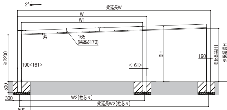
1本梁延長 W>60 正面図
