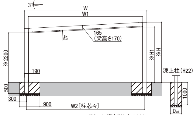
基本・縦2連棟 正面図
