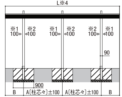
基本(W:33型) 側面図
