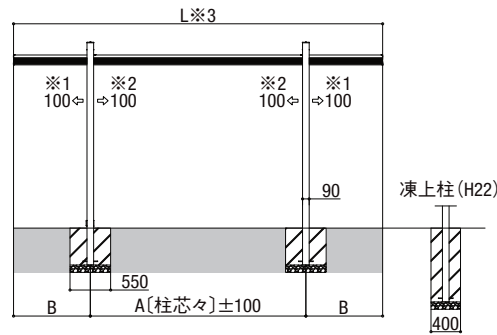
基本(W:30・33型) 側面図
