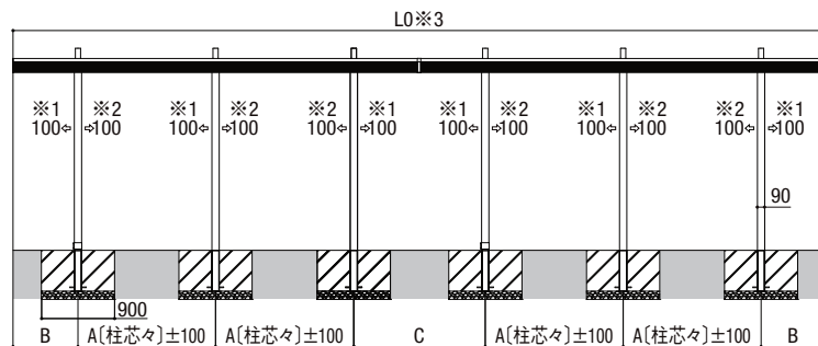
縦2連棟(W:33型) 側面図
