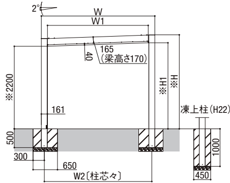
基本・縦2連棟 正面図
