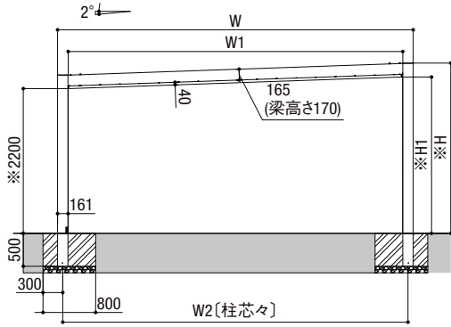
基本・縦2連棟 正面図
