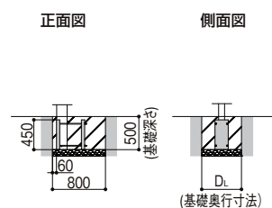
偏心基礎
