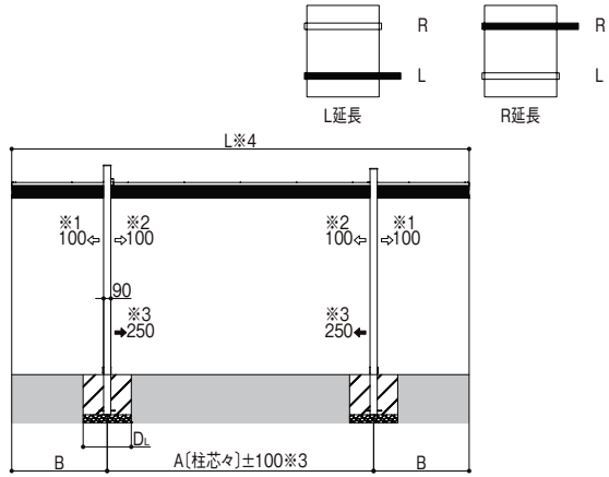
1本梁延長 W≤60 側面図
