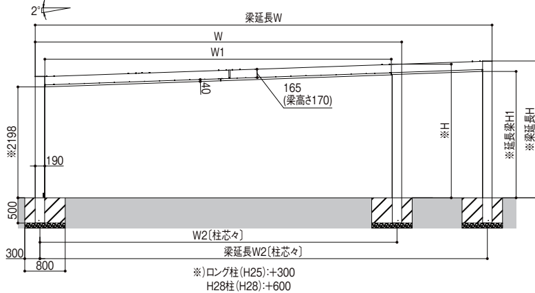
1・2本梁延長 正面図
