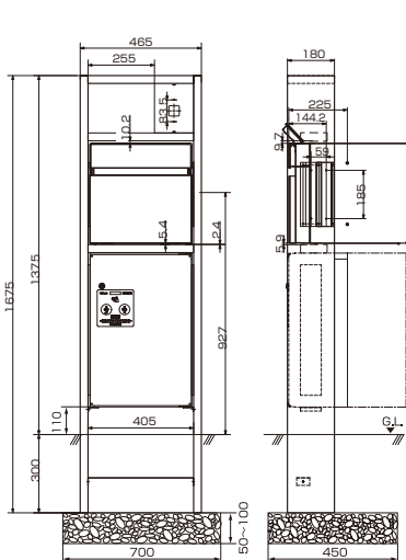
Fタイプ(前入れ・後出し)
