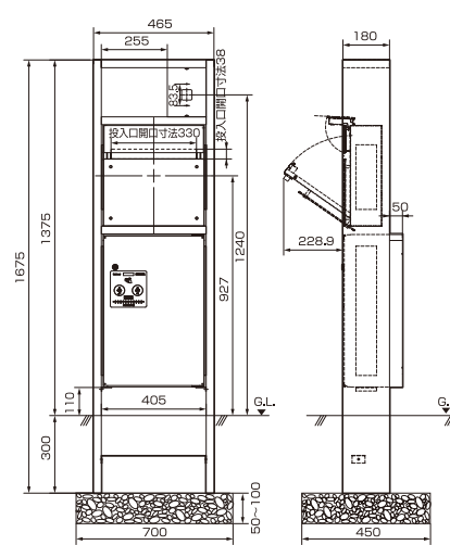
Fタイプ(前入れ・前出し)
