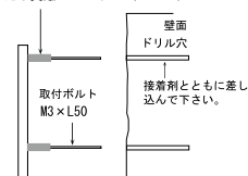
キリモジ円游隼 共通側面図
