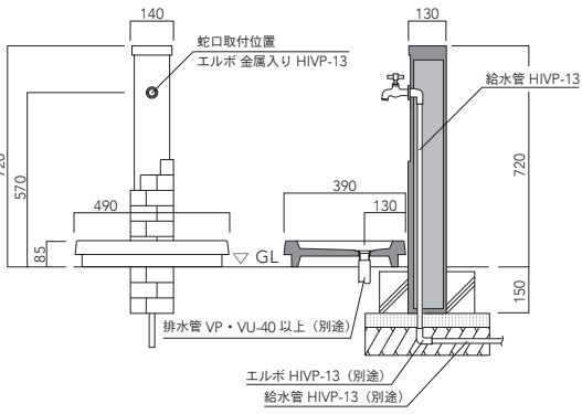
参考施工図
